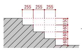
階段断面 S=1/50
