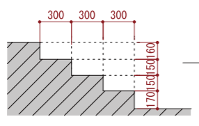
階段断面 S=1/50
