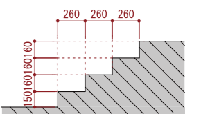
階段断面 S=1/50
